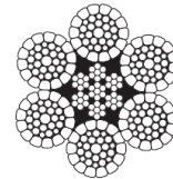
6x36 IWRC Compact
