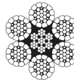
6x31 IWRC Compact
