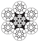
6x19 IWRC Compact
