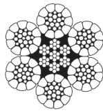
6x26 IWRC Compact
