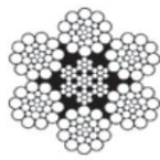
6x26 WS IWRC
